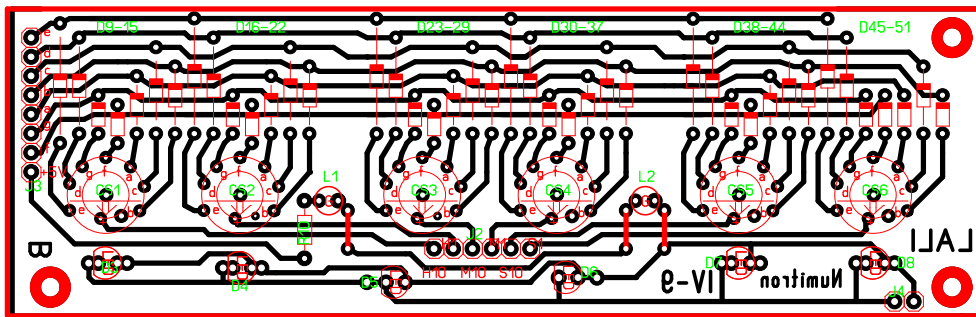
SZABALYZOS, 9 VAC
