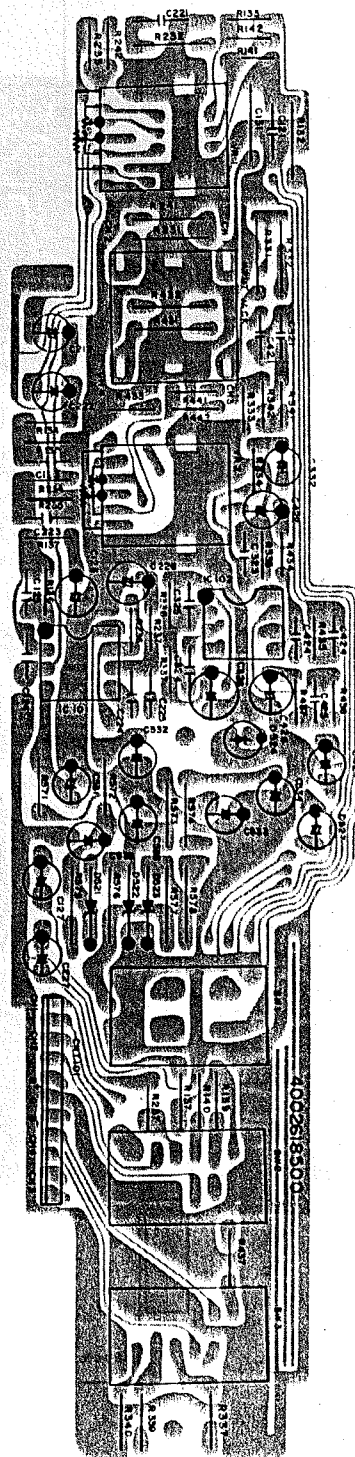
Lötseite Solder Side
