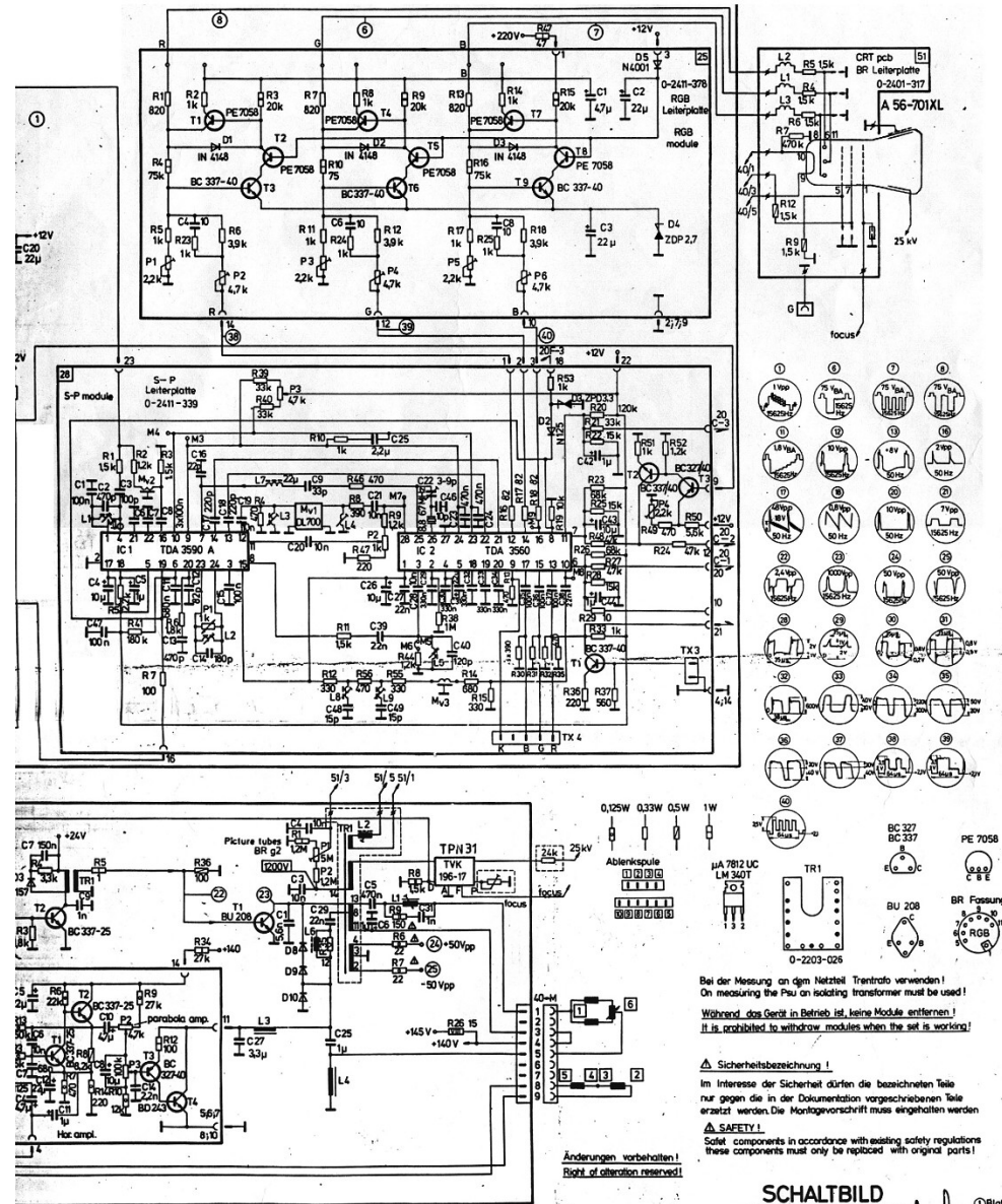
SCHALTBILD CIRCUIT DIAGRAM TS 4377 SP 0-0104-108
