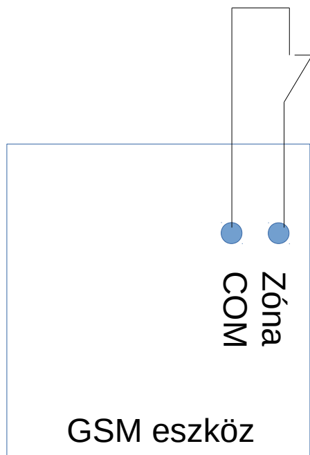
Relé 1 (bontó érintkező)
