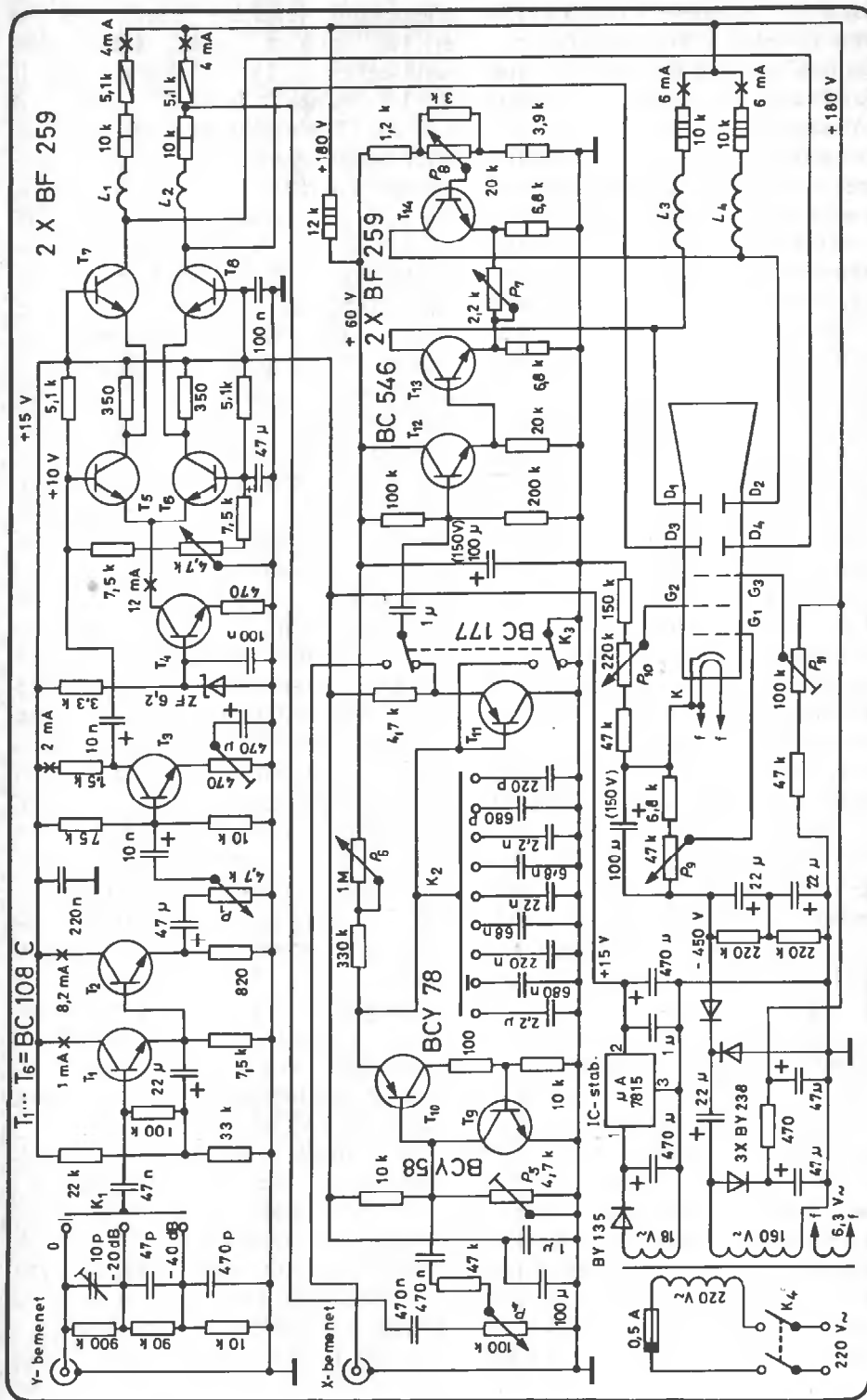
8.3. ábra Tranzisztoros szerviz oscilloszkóp kapcsolási vázlatja
