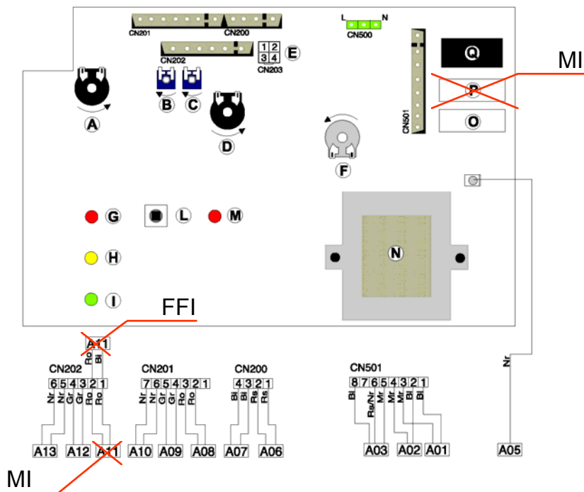
TEC1-TEC2 vezérlőkártyák
