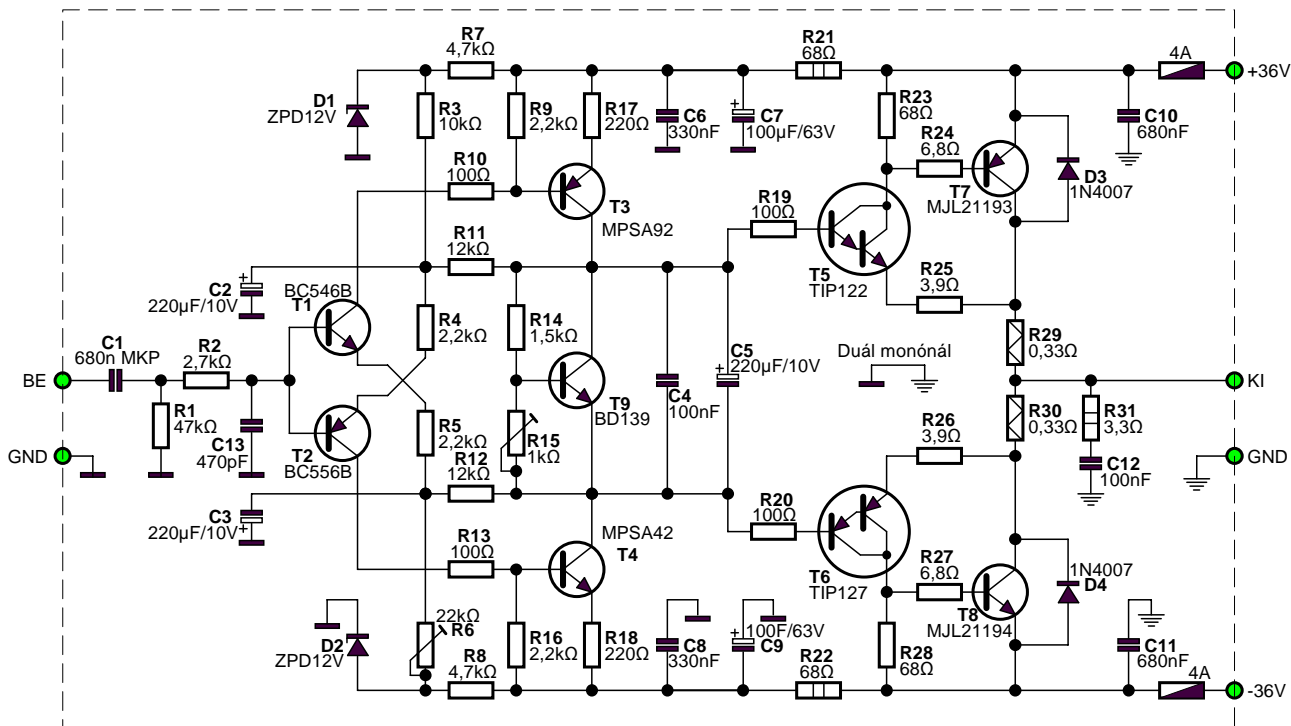
B5 végerősítő (KD mester-től) ALKOTÓ-s ábrájából
