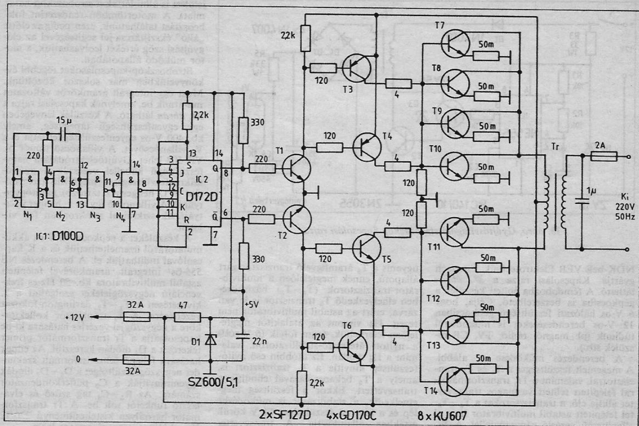
36. ábra. Nagyteljesítményű 12 V/220 V-os transzverter
